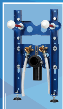
Gomiti flangiati con adduzione dal basso
