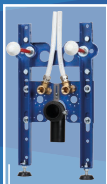
Gomiti flangiati con adduzione dall'alto
