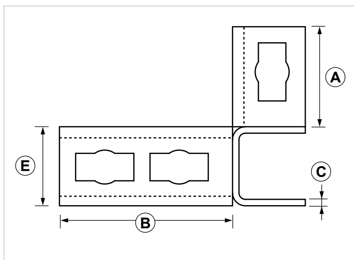
Right angle fitting ANS 90 3D Dx
